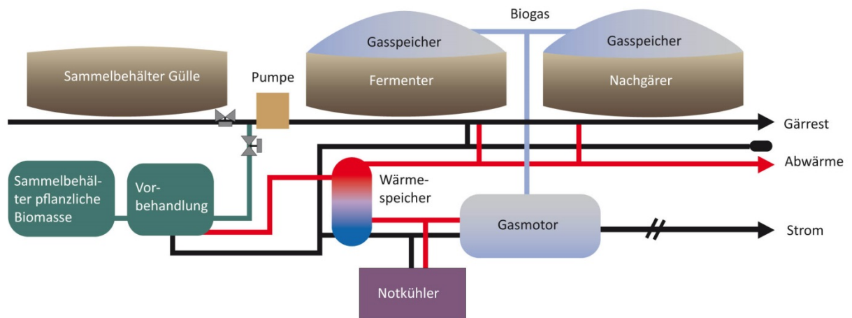
Abbildung 3: Funktionsweise einer Biogasanlage. Grafik: RENAC.
