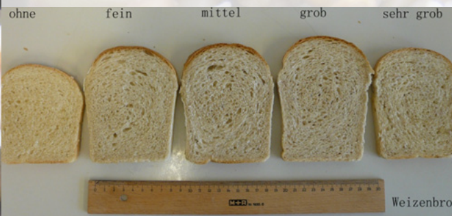
Abbildung 16: Volumenausbeute Weizenbrot Typ 550 2,5 Prozent
