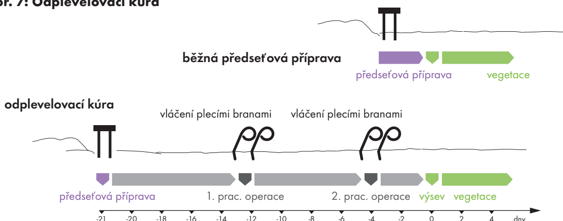
Obr. 7: Odplevelovací kúra
