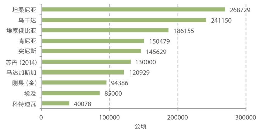
图 46 非洲：2015 年有机面积位列前十位的国家 / 地区 来源：2017 FiBL 调查
