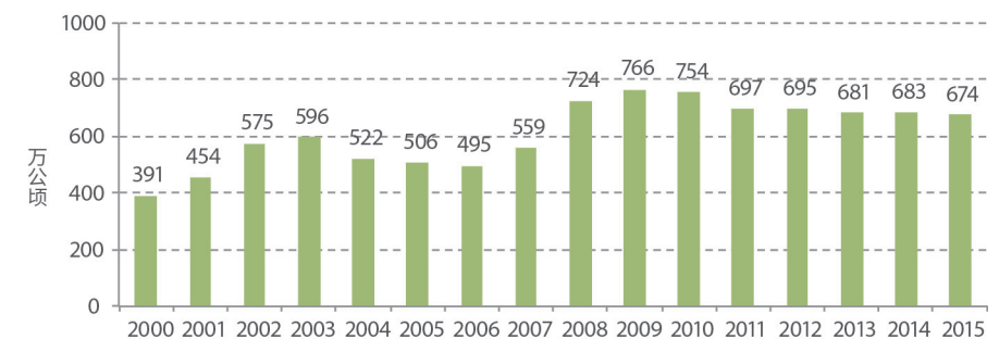
图 81 拉丁美洲和加勒比海地区：2000-2015 年有机农地发展 来源：2002—2017 FiBL-IFOAM-SOEL 调查
