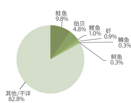
图 27 世界: 有机水产养殖: 2015 年主要品种比例及产量 来源: 2017 FiBL 调查
