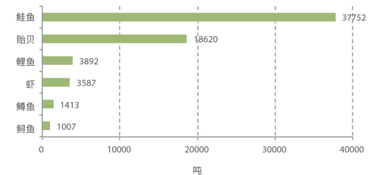
图 27 世界: 有机水产养殖: 2015 年主要品种比例及产量 来源: 2017 FiBL 调查
