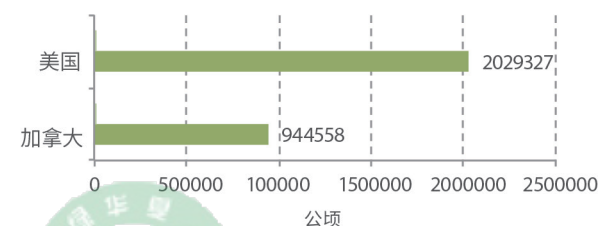
图 86 北美洲: 2015 年美国有机农地面积 来源: OTA 和 USDA, 2016
