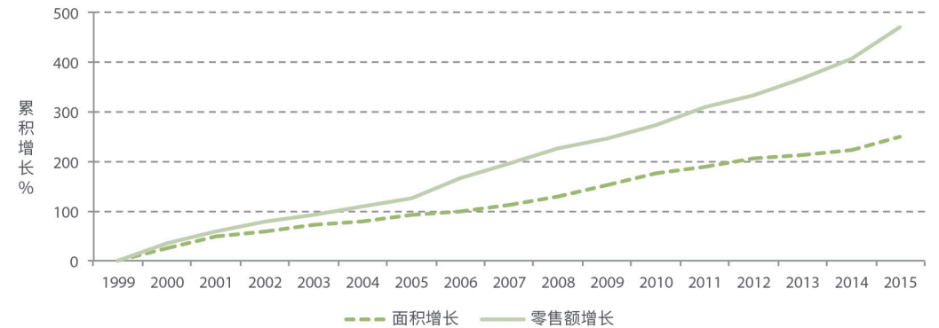
图 55 欧洲: 1999-2015 年有机区域和零售额累积增长情况对比 来源: 2006-2017 FiBL-AMI 调查
