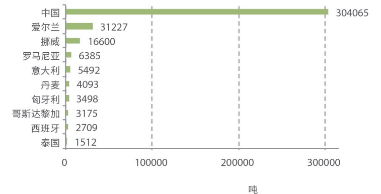
图 26 世界: 有机水产养殖全球分布及产量最大的十个国家 / 地区 来源: 2017 FiBL 调查
